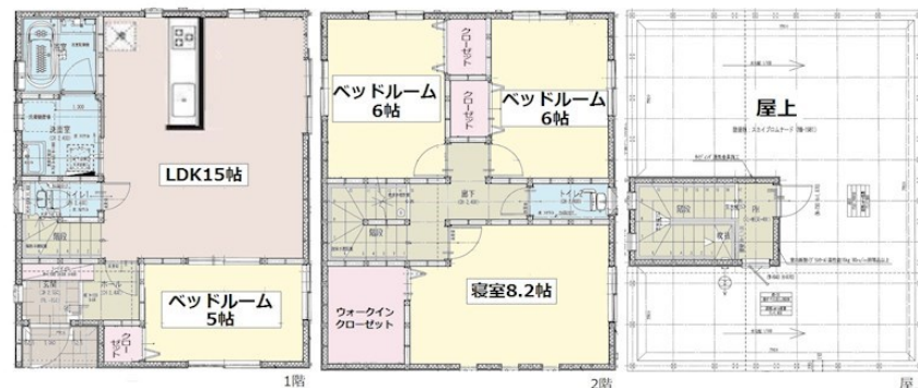
【間取り図】
